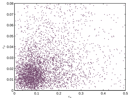
Figure: Raspodela ekscentriciteta za deo uzorka e_v < 0,08 , i e_p < 0,5 koji sadrži 4258 zvezda.
