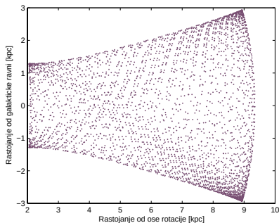
Figure: Oblik i veličina putanje tipične zvezde koja pripada debelom disku Mlečnog puta.
